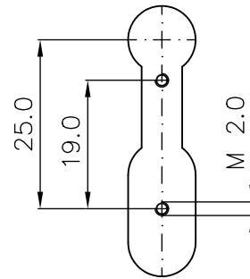
Sonderausführung "19.0" für Zifferblattauflage 2 Gewindebohrungen M 2,0 Abstand 19,0 mm
