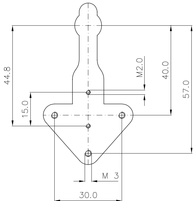
Sonderausführung für Zifferblattauflage und Typenschildmontage
