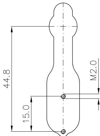
Standardausführung für Typenschildmontage
