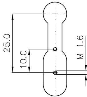
Standardausführung für Zifferblattauflage und Typenschildmontage
