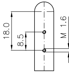
Standardausführung "8,5" für Zifferblattauflage 2 Gewindebohrungen M 1,6 Abstand 8,5 mm
